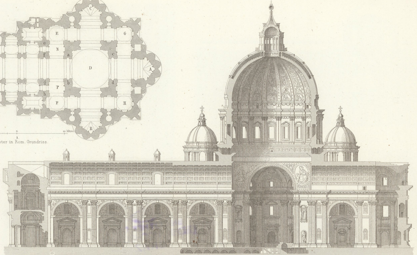
S. Peter in Rom. Längendurchschnitt.
