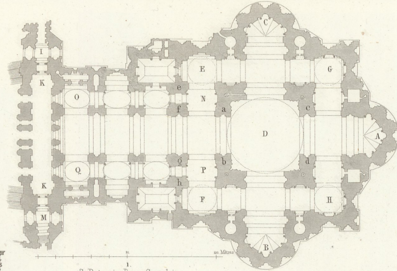
S. Peter in Rom. Grundriss.
