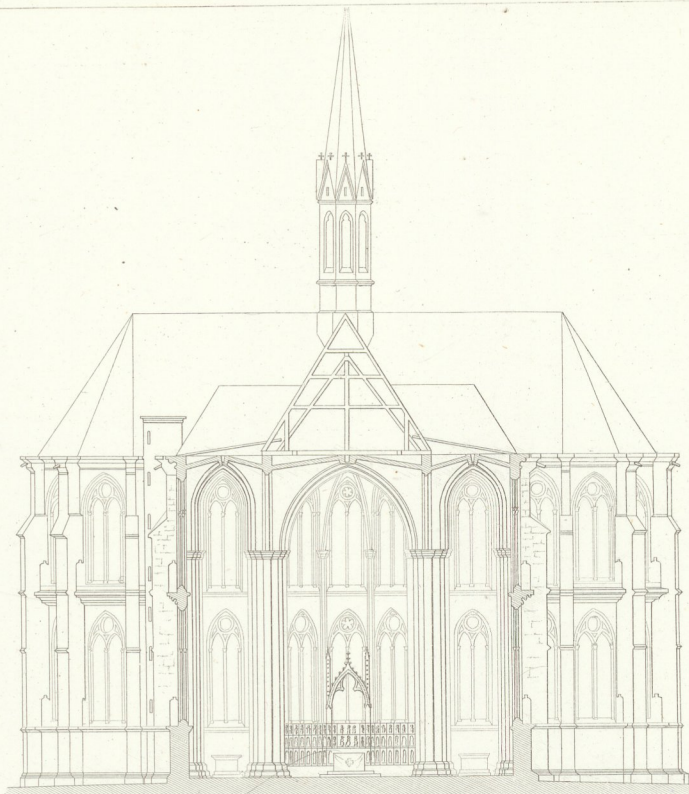
Querschnitt der Elisabethkirche zu Marburg. 6.
