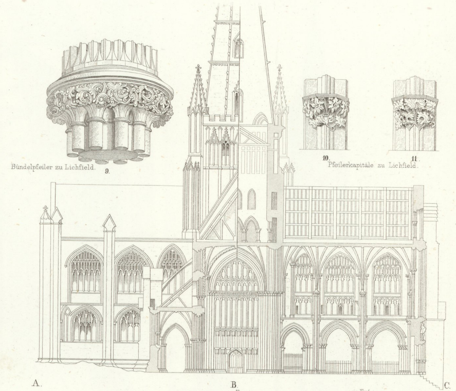
Querschnitt der Cathr. von Lichfield. 8.
