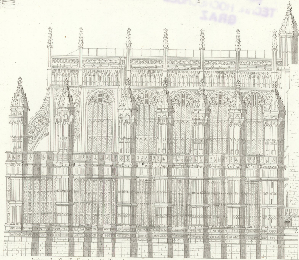
Aufriss der Capelle Heinrichs VII. Westminster. 15.
