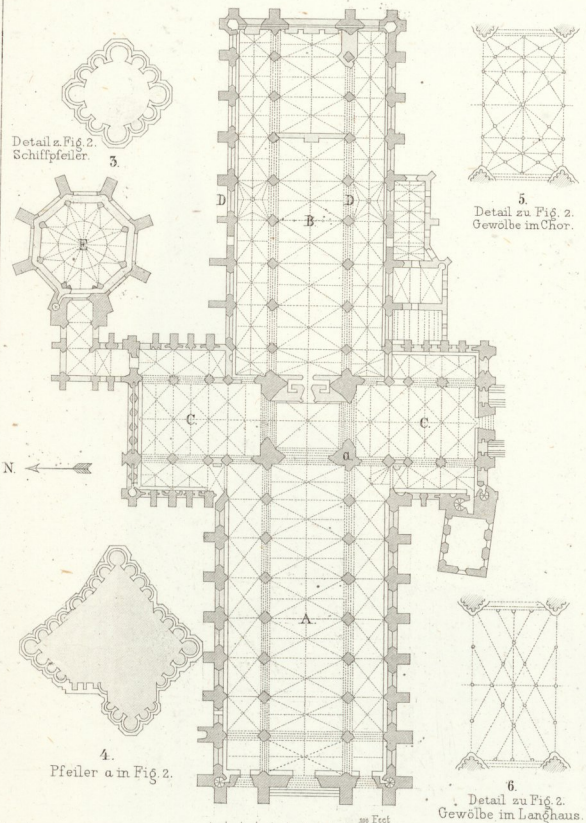
Grundriss der Cathedr. zu York. 2.
