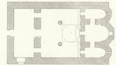
Grundr. zu Fig. 6. 7
