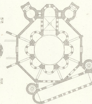
Grundriss von S. Vitale. 9
