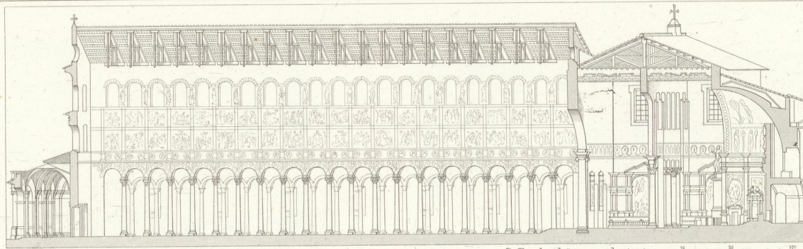
S. Paul. (Längenschnitt)
