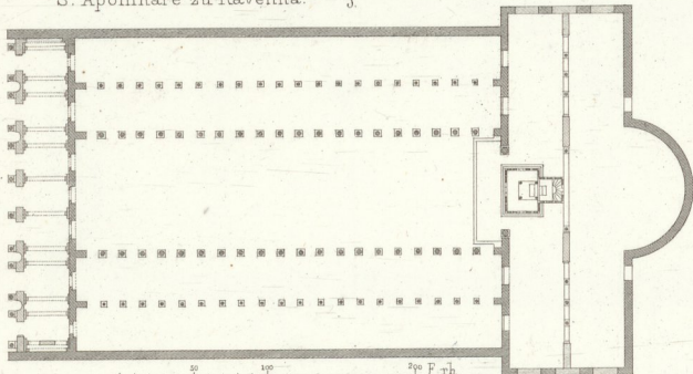
S. Paul. (Grundriss)
