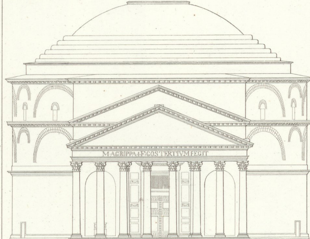
Pantheon. (Aufriss.) 5
