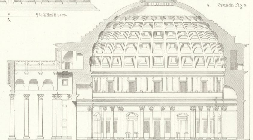
6. Pantheon. (Durchschnitt.)
