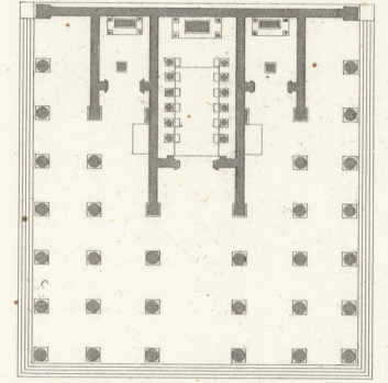
Grundr. zu Fig. 13. 14.
