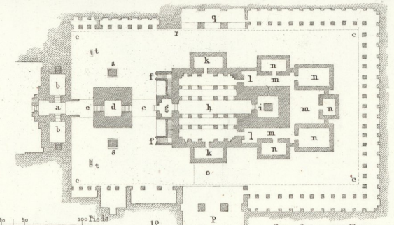
Grundriss zu Fig. 4.
