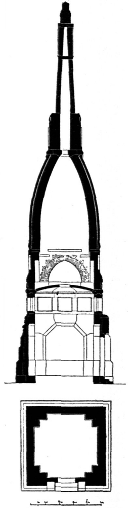
Lotrechter und wagrechter Schnitt.
