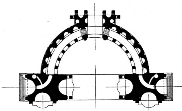
Grundrifs.
