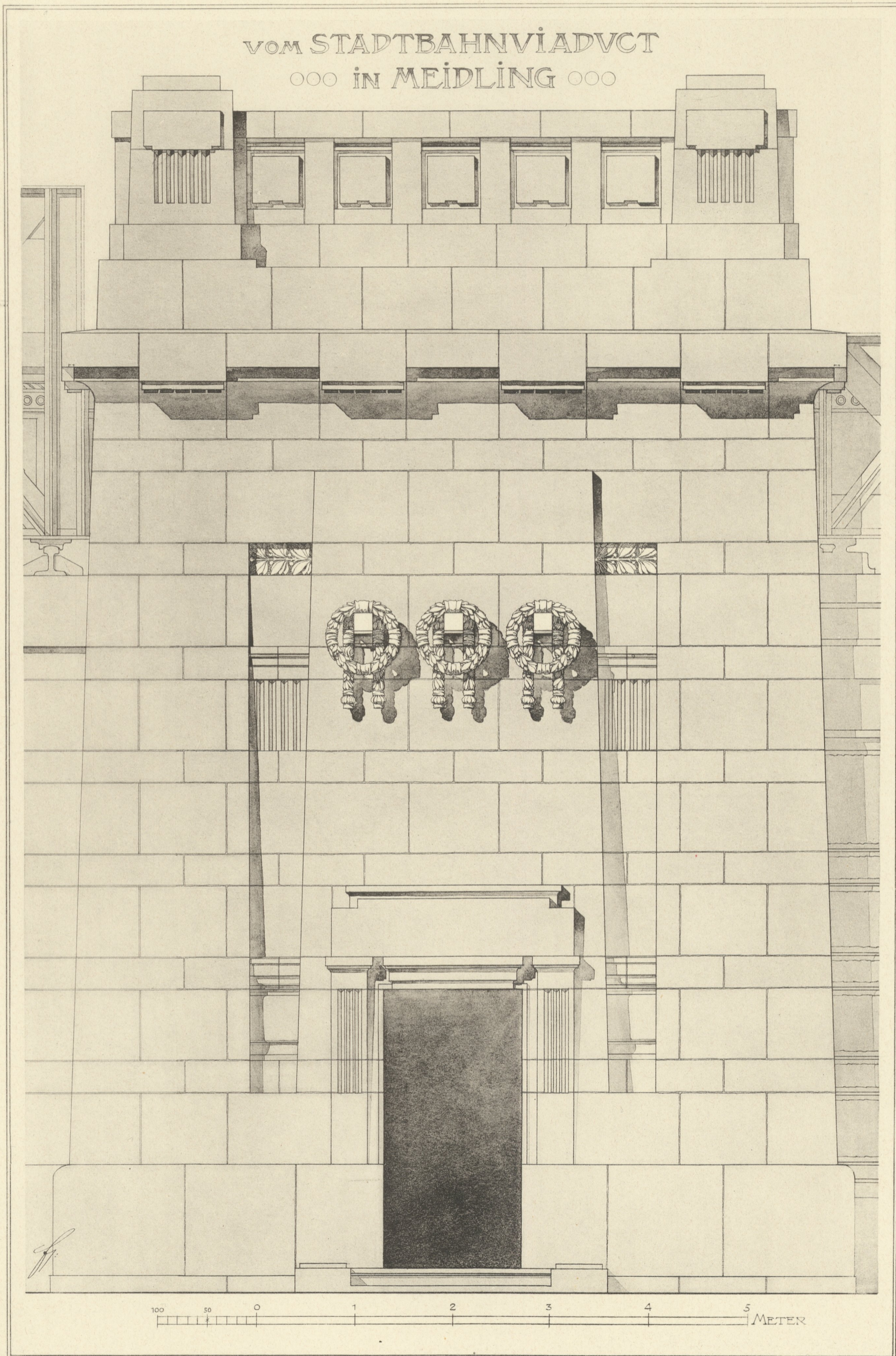
GROSSER BRÜCKENPFILER VOM STADTBAHNVIADUCT IN MEIDLING.
