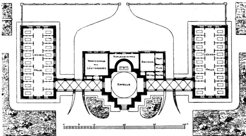
Grundriß.
