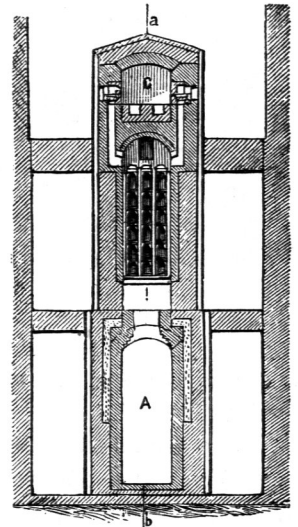
Querschnitt.
