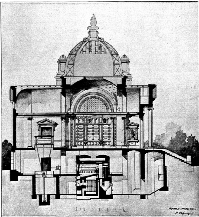
Längenschnitt zu Fig. 269 bis 272 132) ).
