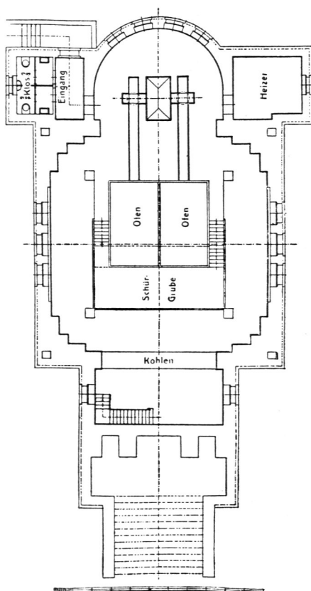
Untergechofs.
