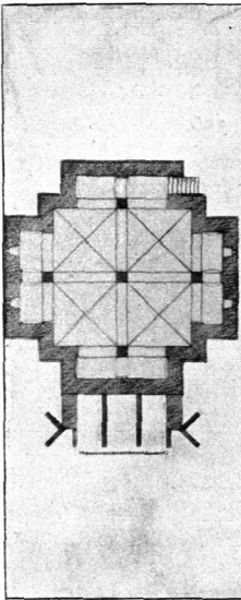
Untergechofs.
