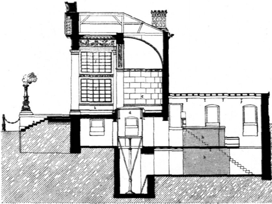
Längenschnitt.
