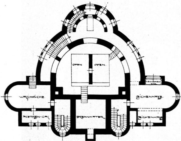
Untergeschoss.
