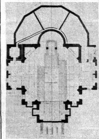
Fig. 258. Untergechofs.
