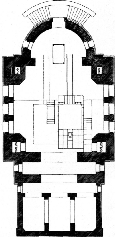
Untergeschoss.
