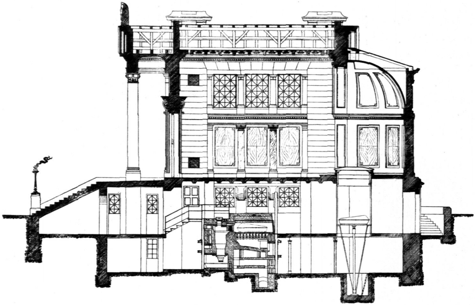
Längenschnitt.
