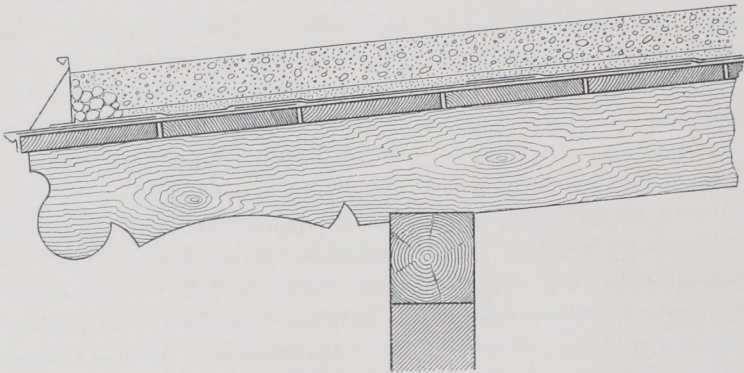
\frac{1}{10} n. Gr.
