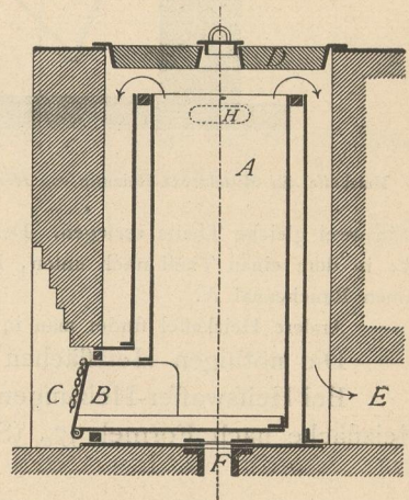
Heizkessel für Niederdruck-Heizung von Hermann Fischer . 1/30 n. Gr.
