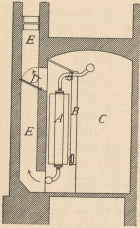
Warmwasserofen für Heizkammern.
