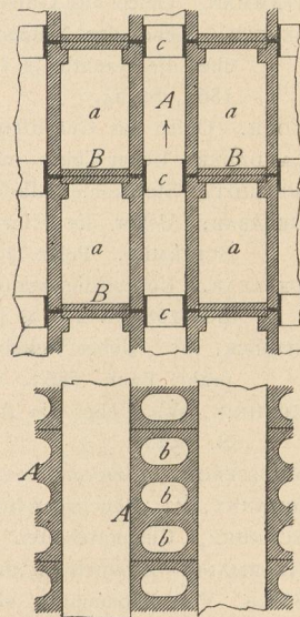
Luftheizungs-Ofen von Gaillard, Haillet & Co. \frac{1}{20} n. Gr.
