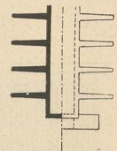
Heizkasten für Warmwasser-Heizung. \frac{1}{10} n. Gr.
