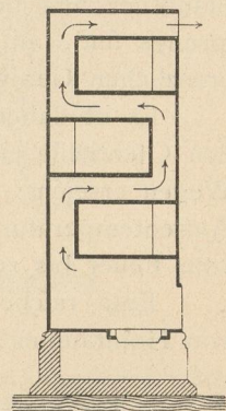
Zickzackofen.
