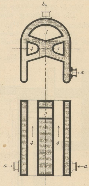
Heizkessel für Niederdruck-Heizung von Hartly & Sugden .
