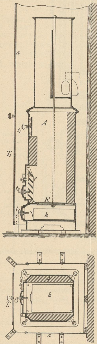
Halbfüllofen.
