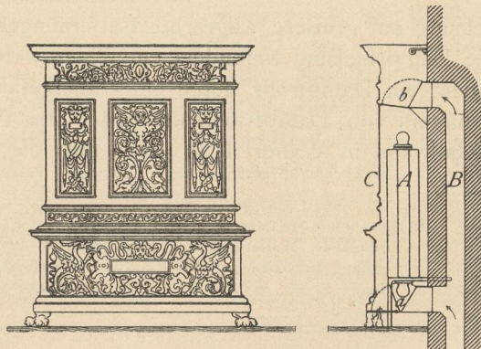
Heizkörper für Warmwasser-Heizung von Aird und Mark in Berlin.
