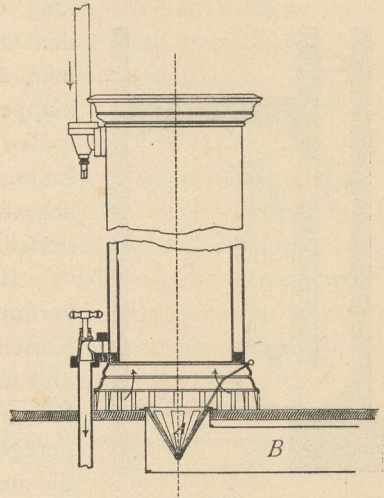
Ofen für Warmwasser-Heizung. \frac{1}{20} n. Gr.
