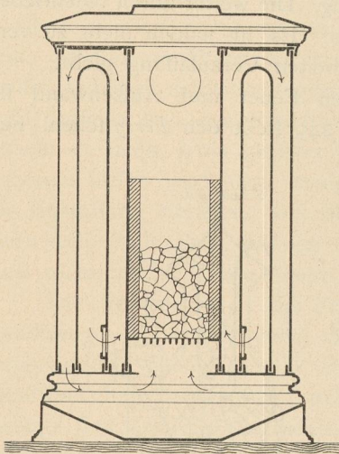
Ofen von Wehrenbold in Lehen a. d. Lippe.
