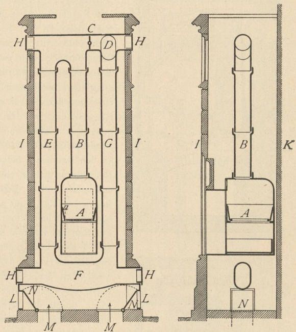
Ofen von Rafsch . \frac{1}{35} n. Gr.
