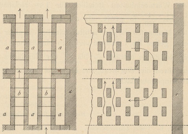
Luftheizungs-Ofen von Wiman . \frac{1}{30} n. Gr.
