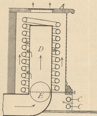
Wärmestrahler für Hochdruck-Heizung. 1/20 n. Gr.
