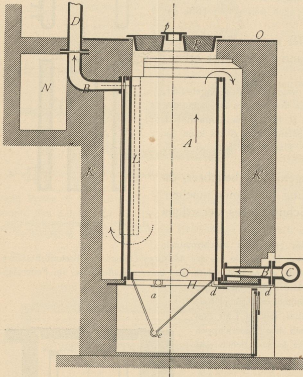
Heizkessel für Mitteldruck-Heizung von Hermann Fischer. \frac{1}{30} n. Gr.
