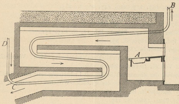
Heizapparat für Hochdruck-Heizung von Schinz. \frac{1}{50} n. Gr.
