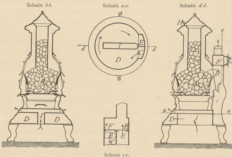
Schnitt ee. Perry's amerikanischer Ofen.
