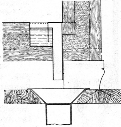
Abflufs aus Eisschränken. — \frac{1}{5} n. Gr.
