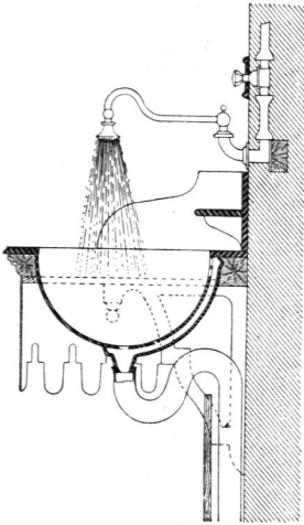
Wach-Toilette mit Schwenkhahn und Brause. — 1/20 n. Gr.
