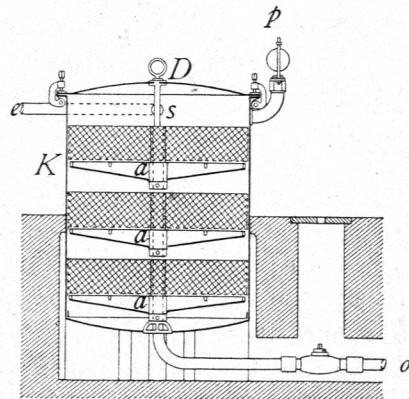
Kartoffelsieder in der Küche der Irrenanstalt zu Neustadt-Eberswalde 12) . — \frac{1}{25} n. Gr.
