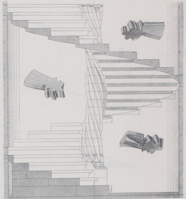
Treppe im Schloß zu Tübingen 72) . 1/50 n. Gr.
