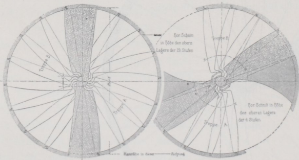
Treppe in der Georgs-Kirche zu Nördlingen 76) . 1/50 n. Gr.
