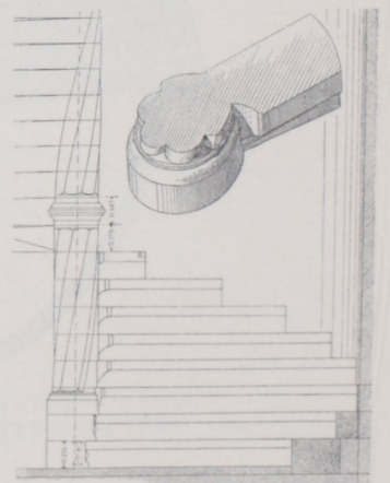
Von der Treppe im Schloßchen zu Stammheim 75) . 1/50 n. Gr.
