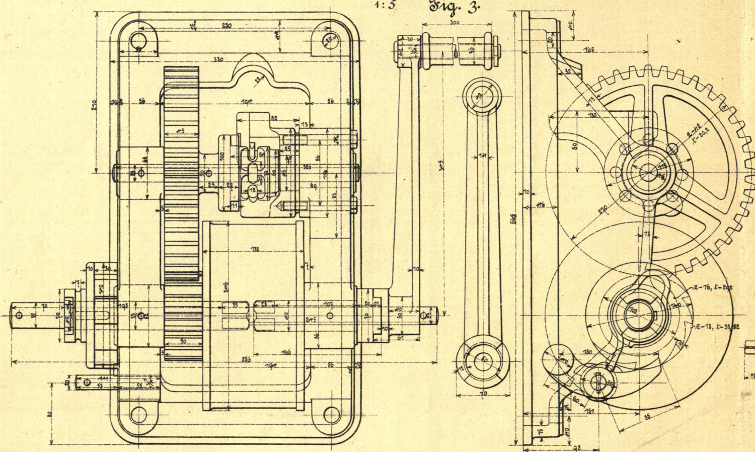
Ketten-Wandwinde von 300 kg Tragkr. mit Sicherheitskurbel und Schleuderbremse v. Buegler, Hansen & Co., Gotha
