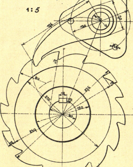
Fig. 8. 1:5
