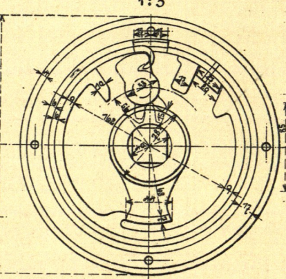
Fig. 12. 1:5
