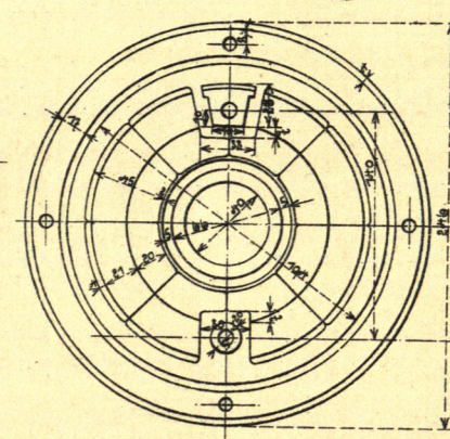
Fig. 9. 1:5
