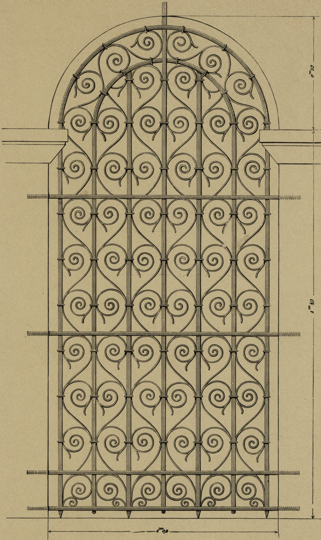
Schmiedeeiserne Vergitterung eines Bogenfensters; entworfen von Architect Bénard in Paris.
