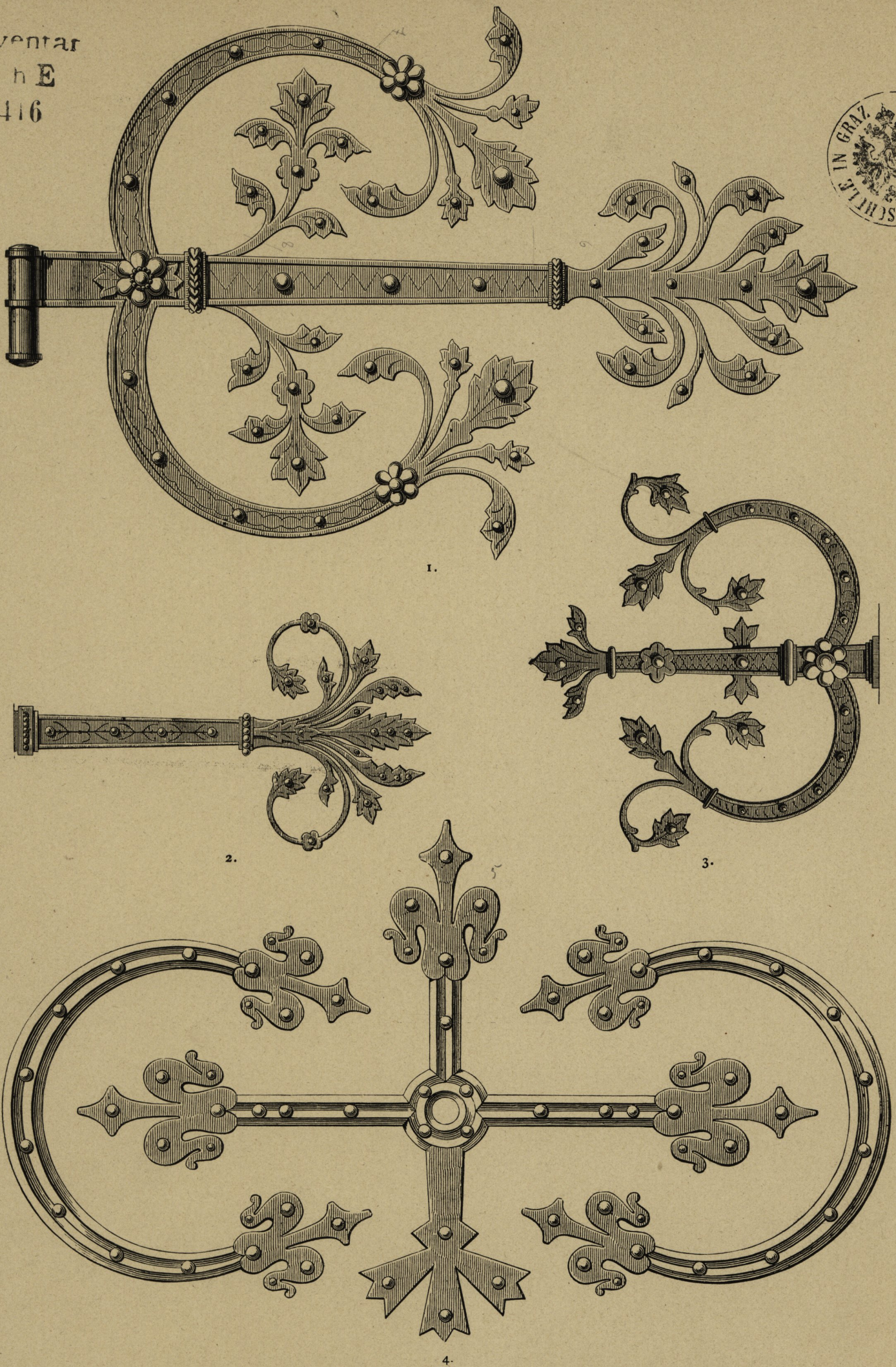
1—3. Thürbeschläge an der protestantischen Kirche in Brünn; entworfen von Oberbaurath Professor Baron von Ferstel, ausgeführt von Schlosser Nowitzky. 4. Thürbeschläge aus der Klosterkirche zu Maulbronn (Württemberg). 15. Jahrhundert.
