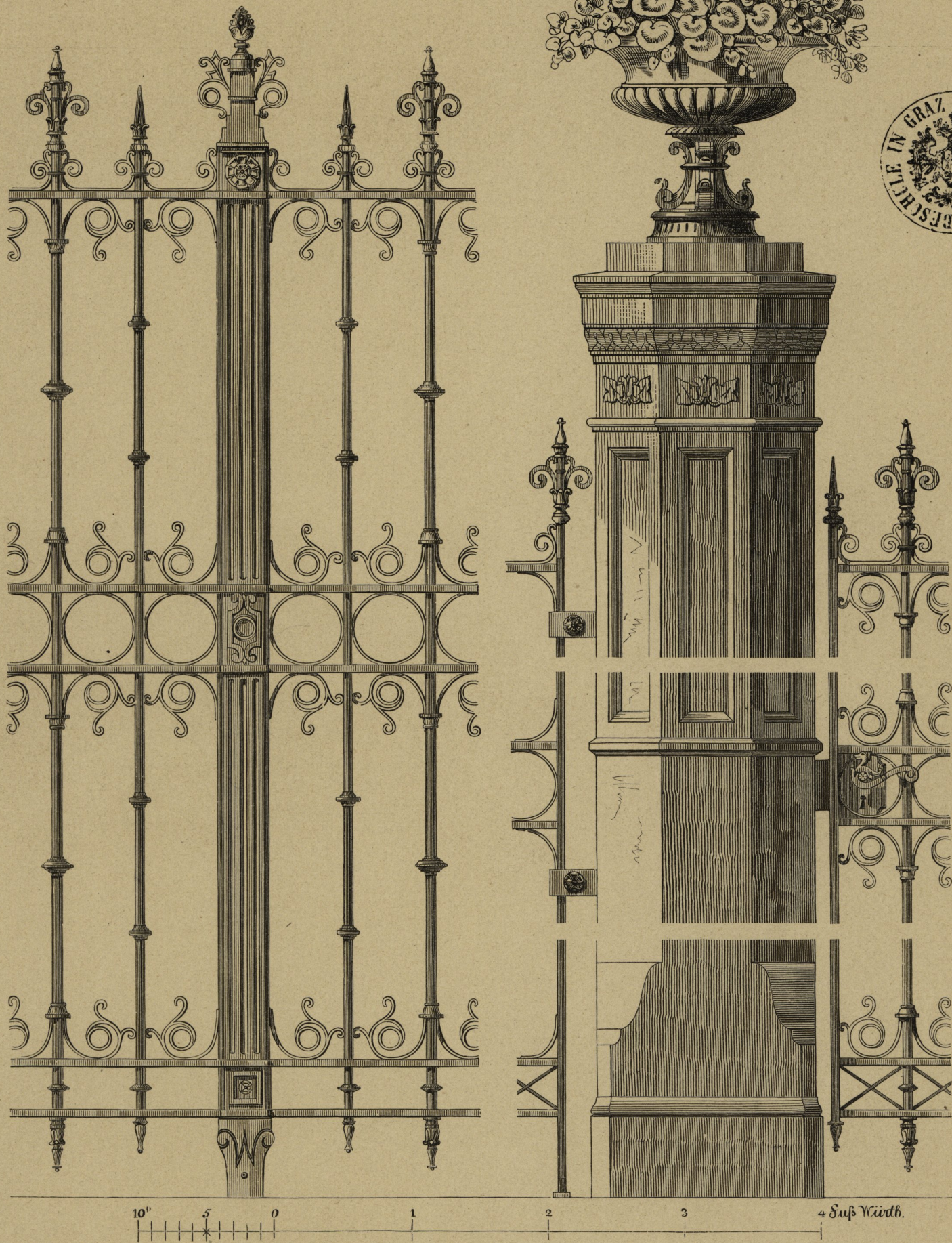
Details zu dem auf Tafel 48 (1.) abgebildeten Gitterthor.
