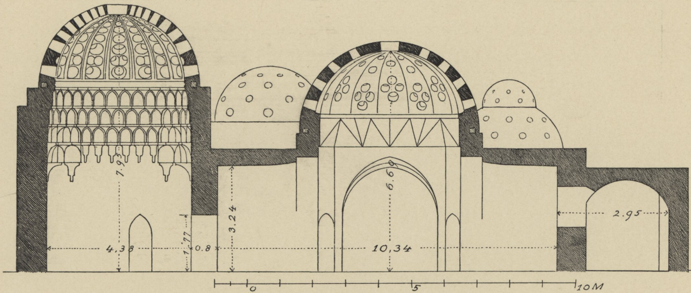
Fig. 52 Schnitt durch das Badhaus.
