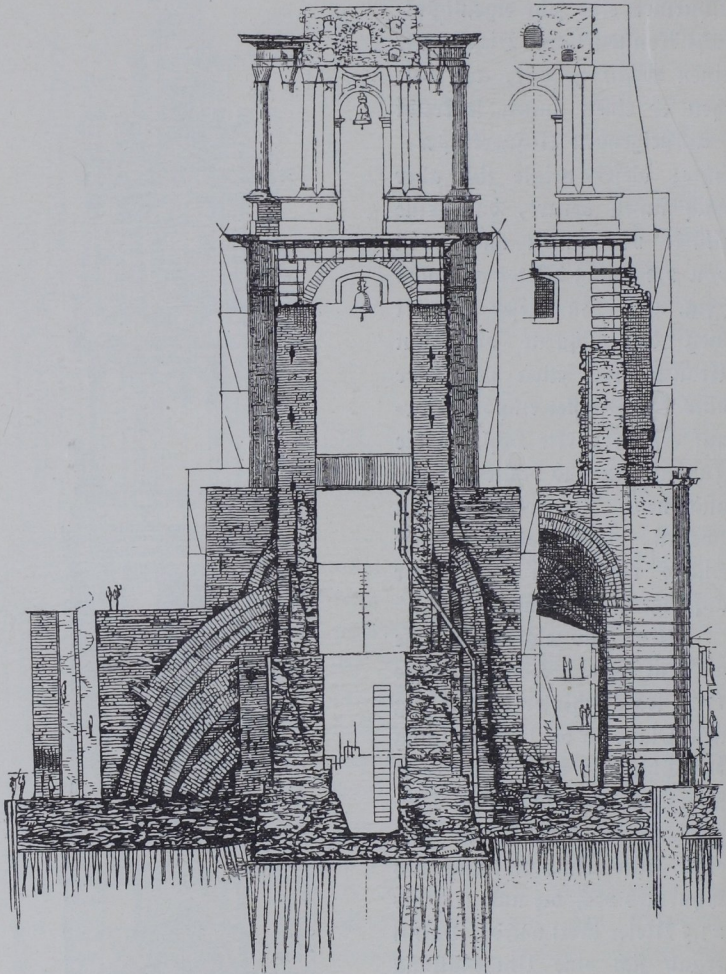
Fig. 48. Broebes' Skizze zum Bau des Münzthurmes.
