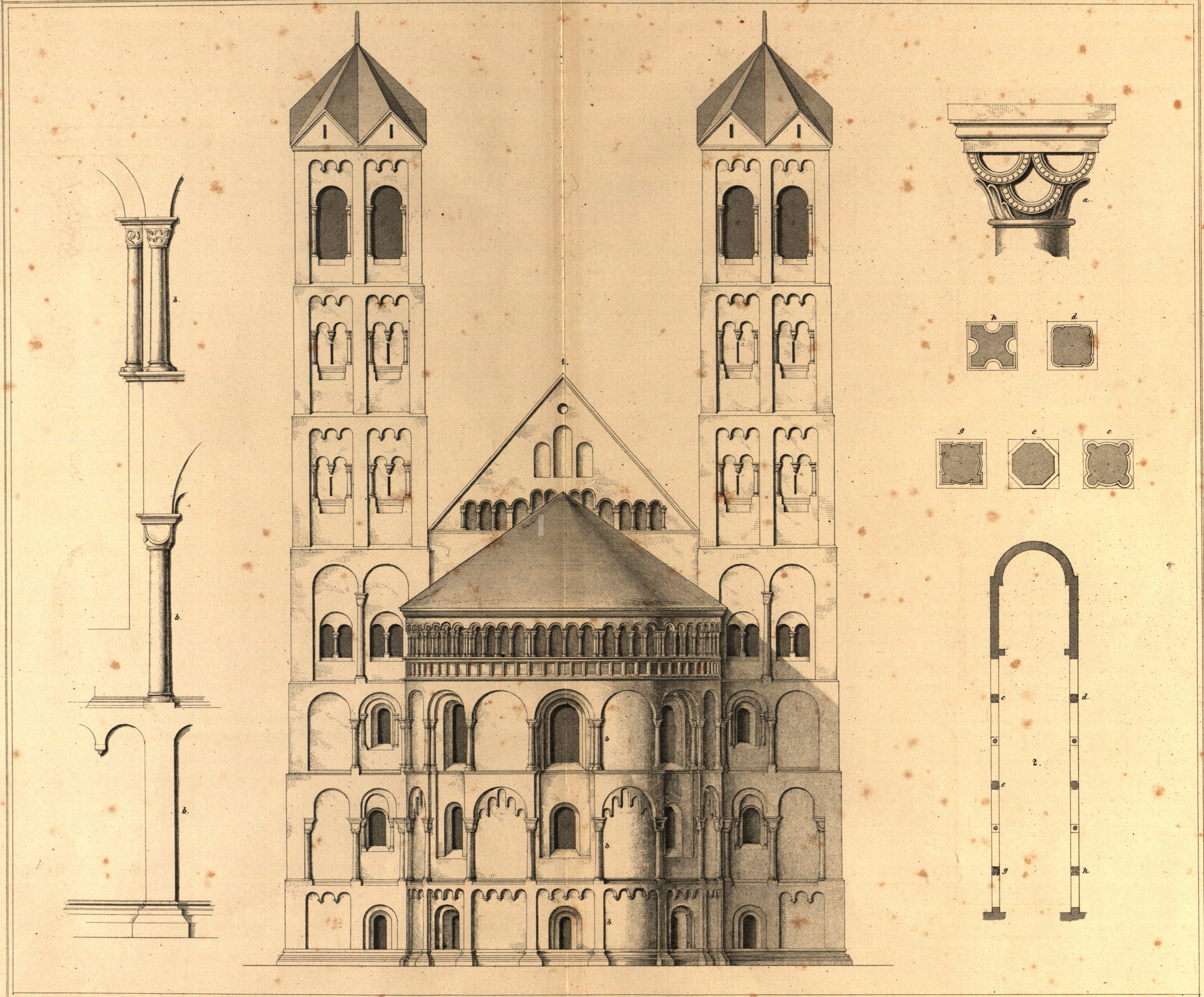
1. Die Ostseite der Kirche St. Gereon zu Cöln. 2. Grundriß des Schiffes der St. Nicolai Kirche zu Eisenach. Während das Hauptschiff der Halberstädter Frauenkirche auf Pfeilern, das von Kaulinzelle auf Säulen ruht, sehen wir im Grundriß 2. Pfeiler und Säulen abwechseln. Jeder der sechs Pfeiler hat eine andere Form: a ist ein Säulen Capital dieser Kirche. Der Chor bei 1. hat Verwandtschaft mit dem von St. Martin, während die Thürme vierseitig bleiben. Die Thurmdächer, an jeder Seite mit 2. Giebeln, sind weitere Entwicklung der Thurmdächer von der Halberstädter Kirche 1040 - 1050.
