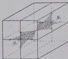
Fig. 511. Dispersion r \perp bl .
