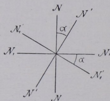
Fig. 470. Zirkularpolarisation. (Drehung der Schwingungsebene linear polarisierten Lichtes.)
