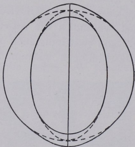
Fig. 469. Strahlengeschwindigkeitsflächen eines zirkular polarisierenden optisch einachsigen Kristalls.
