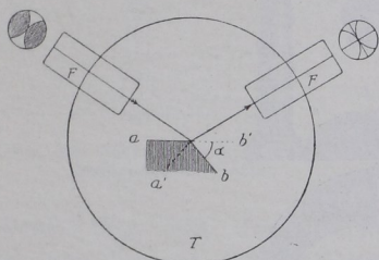
Fig. 343. Schema des Reflexionsgoniometers.
