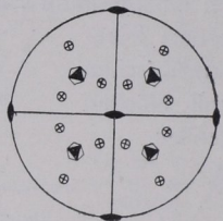
Fig. 243. Allgemeines dyakisdodekaedrisches Bauschema.
