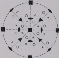
Fig. 241. Allgemeines pentagonikositetraedrisches Bauschema.
