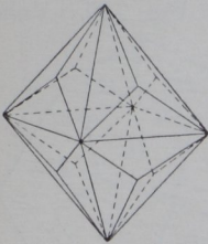
Fig. 230. Ein Pyramidenoktaeder.
