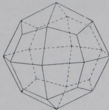
Fig. 231. Ein Ikositetraeder.
