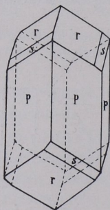
Fig. 164. Dioptas.
