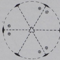
Fig. 152. Erzeugende Symmetrie der ditrigonal-bipyramidalen Klasse ( 3s ).
