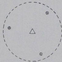
Fig. 154. Erzeugende Symmetrie der trigonal-bipyramidalen Klasse ( 3\rho ).
