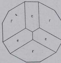
Fig. 158. Eisenglanz.
