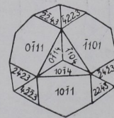
Fig. 159. Eisenglanz.
