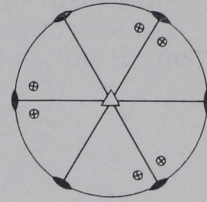
Fig. 153. Allgemeines ditrigonal-bipyramidales Bauschema.
