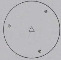
Fig. 155. Allgemeines trigonal-bipyramidales Bauschema.
