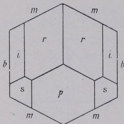
Fig. 101. Hornblende (Kopfbild).
