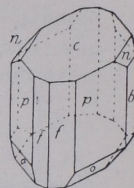
Fig. 104. Realgar.
