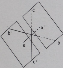
Fig. 79. Pinakoid 1. Art.
