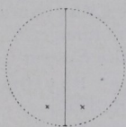
Fig. 60. Pedion. Fig. 61. Pinakoid. Fig. 62. Sphenoid. Fig. 63. Doma. Fig. 64. Prisma.
