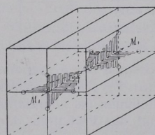
Fig. 509. Geneigte Dispersion. Fig. 510. Geneigte Dispersion. Fig. 511. Dispersion r \perp bl .
