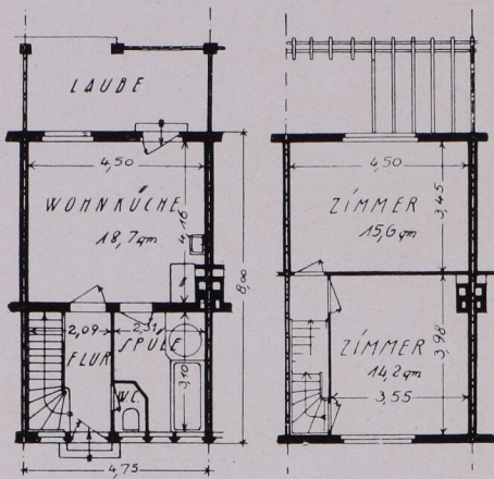
Erdgeschoß
