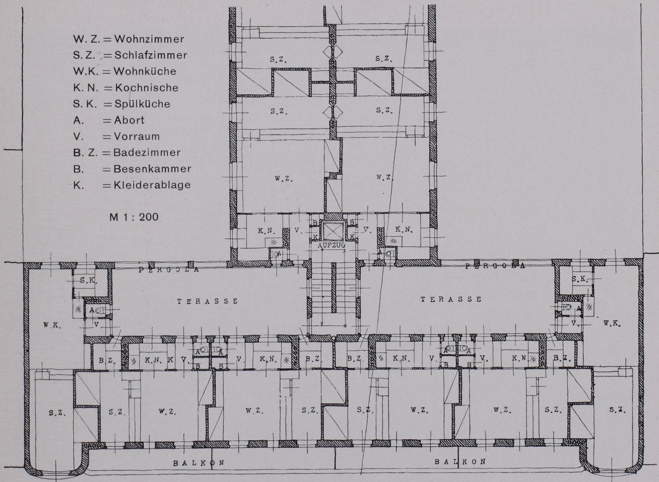
Grundelemente der Kleinwohnung. Entwurf für Wien XIX
