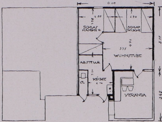
Grundriß zum Sommerhaus in Pichelswerder
