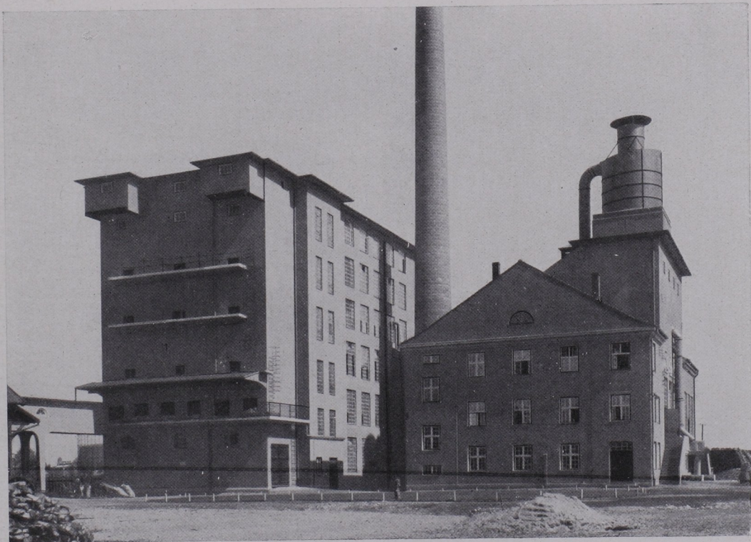
Hofseite mit Verwaltungsgebäude und Maschinen- u. Kesselhaus Fabrikanlage in Königsberg Architekt Kurt Frick, Königsberg
