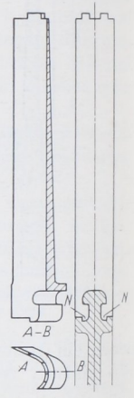
Abb. 2249. Schaufelbefestigung der Bergmann-Werke Berlin.
