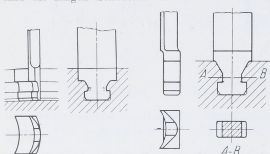
Abb. 2247. Verstärkter Hammerfuß.
