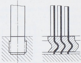
Abb. 2251. Befestigung der Brunner Maschinenfabrik.
