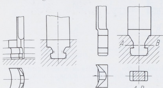
Abb. 2247. Verstärkter Hammerfuß.
