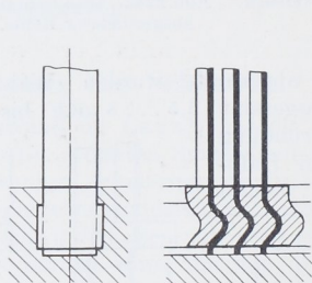
Abb. 2251. Befestigung der Brünner Maschinenfabrik.
