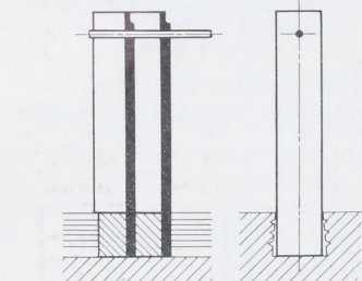
Abb. 2250. Ältere Schaufelbefestigung nach Parsons.
