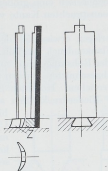
Abb. 2239. Schaufelbefestigung mittels Schwalbenschwanzes.
