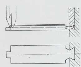
Abb. 2241. Schlagbiegeversuch an Schaufeln.
