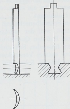
Abb. 2240. Gegenschwalbenschwanz.
