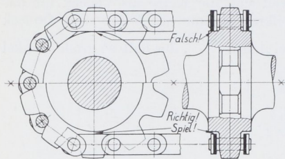
Abb. 2177. Richtige und falsche Ausbildung der Kettenräder.
