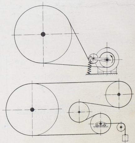
Abb. 2009 und 2010. Riemen- oder Seiltriebe mit Spannrollen.
