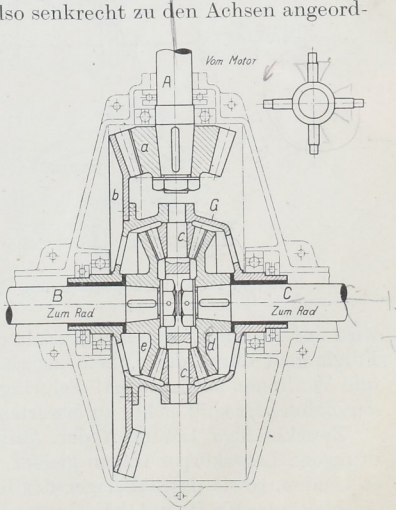
Abb. 1952. Kegelrad- und Ausgleichgetriebe an Kraftwagen.
