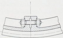
Abb. 1902. Kranzverbindung.
